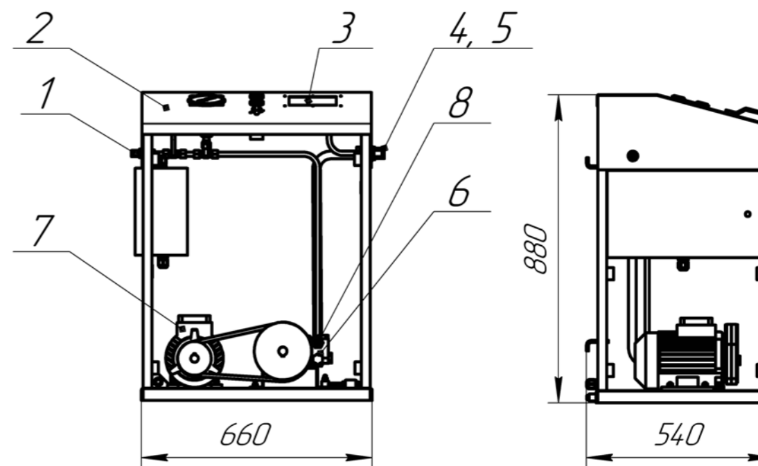
Станция зарядная углекислотная СЗУ-500 (СЗУ-500Д). Габаритный чертеж.
