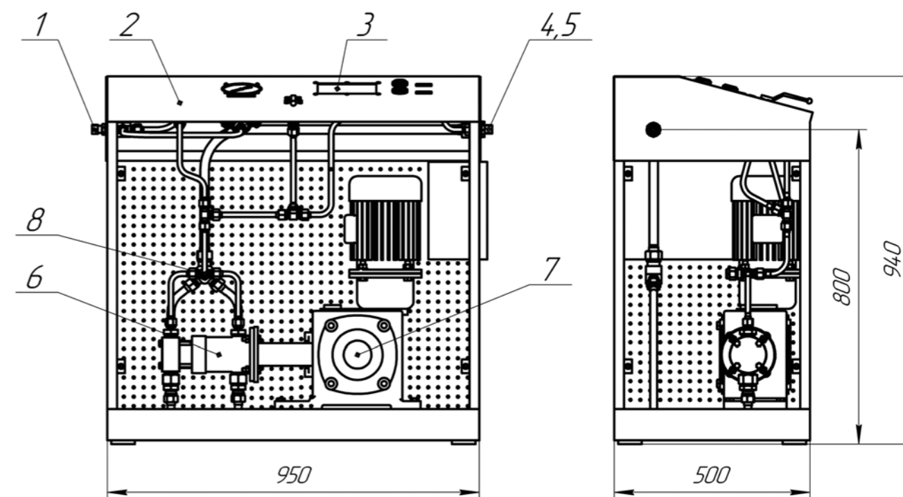
Станция зарядная углекислотная СЗУ-800 (СЗУ-800Д). Габаритный чертеж.
